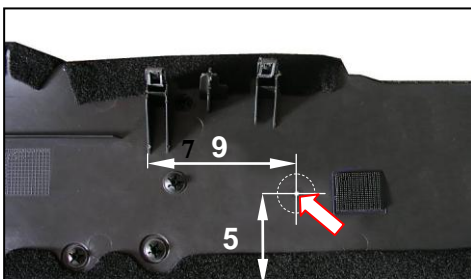
Разметить отверстие в боковой крышке под корпус замка
