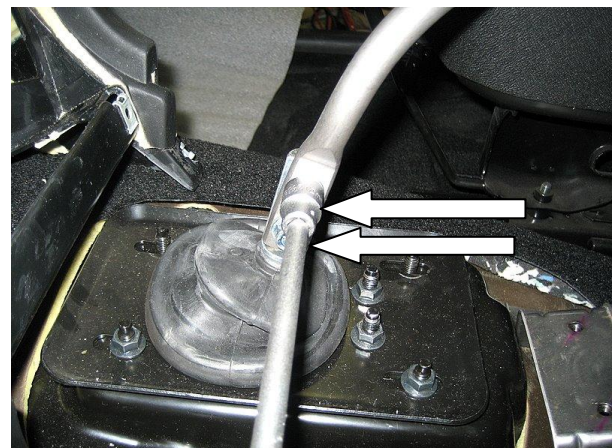
Открутить 2 штатных болта рычага переключения передач
