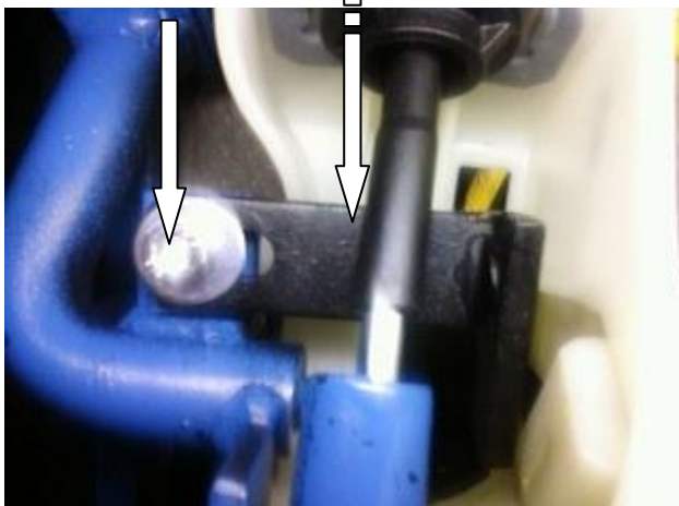
Установить защиту ригеля на лапку замка, закрутить болт
