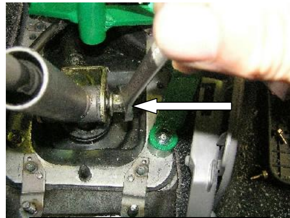
Открутить штатную гайку рычага переключения передач
