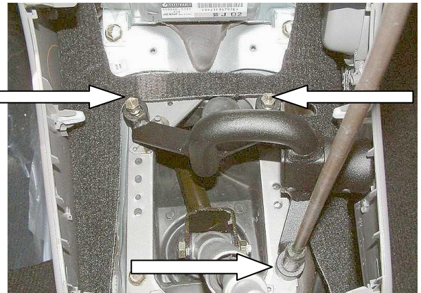
Установить замок, закрутить 3 срывных болта
