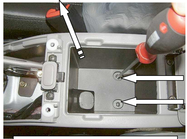
Поднять подлокотник, открутить 2 самореза, снять консоль
