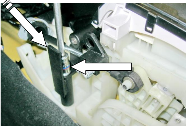
Установить защиту ригеля, закрутить болт
