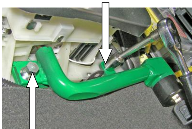
Установить замок на пластину-переходник
