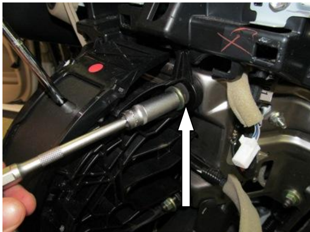
Открутить гайку
