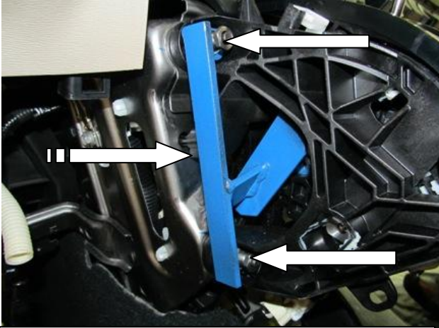
Установить защиту, закрутить 2 гайки
