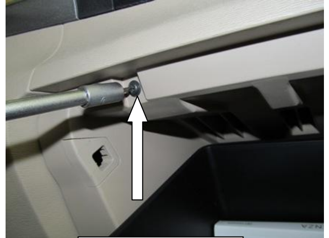
Открутить саморез
