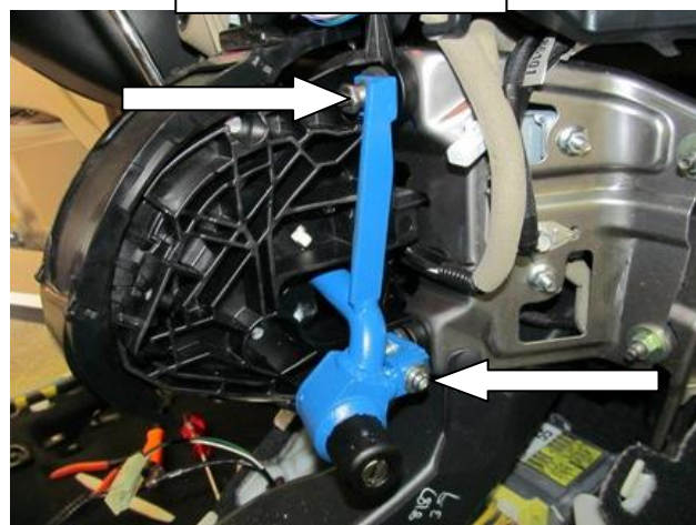
Установить замок на деталь- переходник, закрутить болт и гайку
