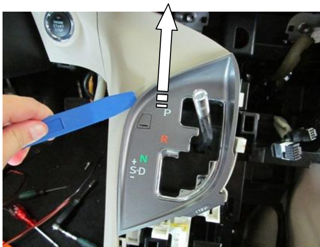
Снять декоративную панель
