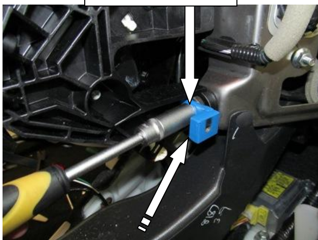
Установить деталь- переходник, закрутить гайку
