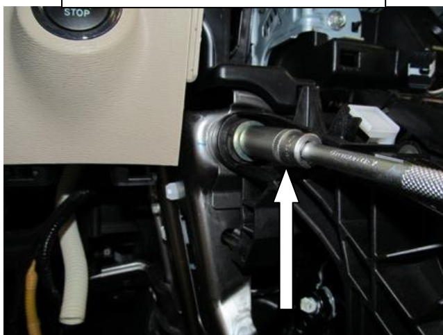
Открутить гайку
